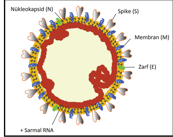
Şekil 1. Coronavirüslerin şematik gösterimleri (6). S, M ve E proteinleri lipid katmanı içerisinde coronavirüslerin zarf yapısını oluşturmaktadır. N proteinini genomik viral RNA bağlar.
